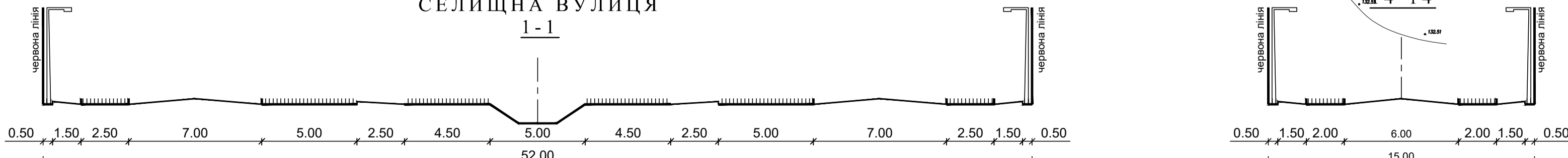
ПОПЕРЕЧНИЙ ПРОФІЛЬ ВУЛИЦЬ СЕЛИЩНА ВУЛИЦЯ 1-1
